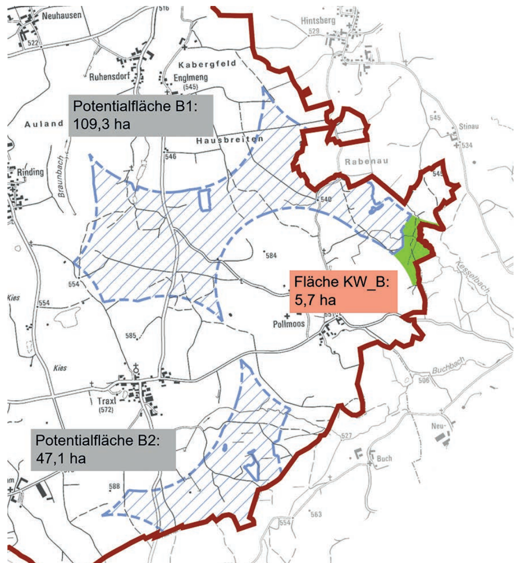
Abbildung 2 ▲ und 3 ▼: Planung Konzentrationszonen (ohne Maßstab, Entwurf 25.07.2023 Plan Nr. 1347-3-2)
